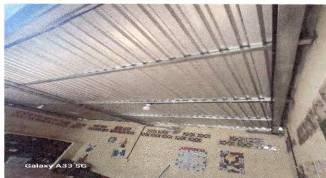
Foto 1 : Cubierta de lámina y estructura de techo: Sustitución de lámina acanalada por lámina troquelada y sustitución de estructura de soporte de metal, en módulo 1 en aulas.
